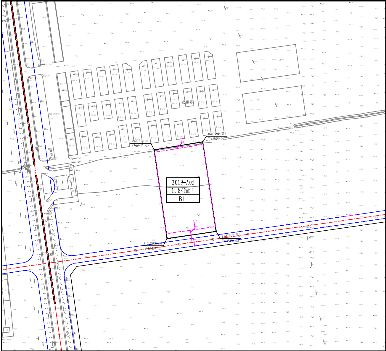
2019-A05地块(迎宾大道东侧)商业用地控详规划图
